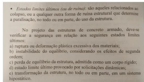
Figura 2 - Requisitos para ELU segundo José Milton de Araújo - referenciados pela ABNT NBR 6118/2014
