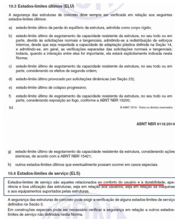
Figura 1 - Requisitos para ELU e ELS apresentados pela ABNT NBR 6118/2014
