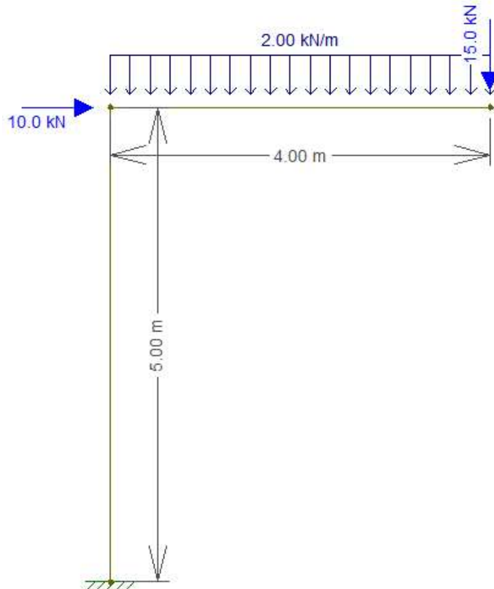
Figura 1: Pórtico submetido a carregamentos
