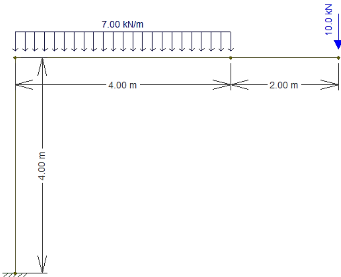
Figura 1 – Pórtico submetido a carregamentos
