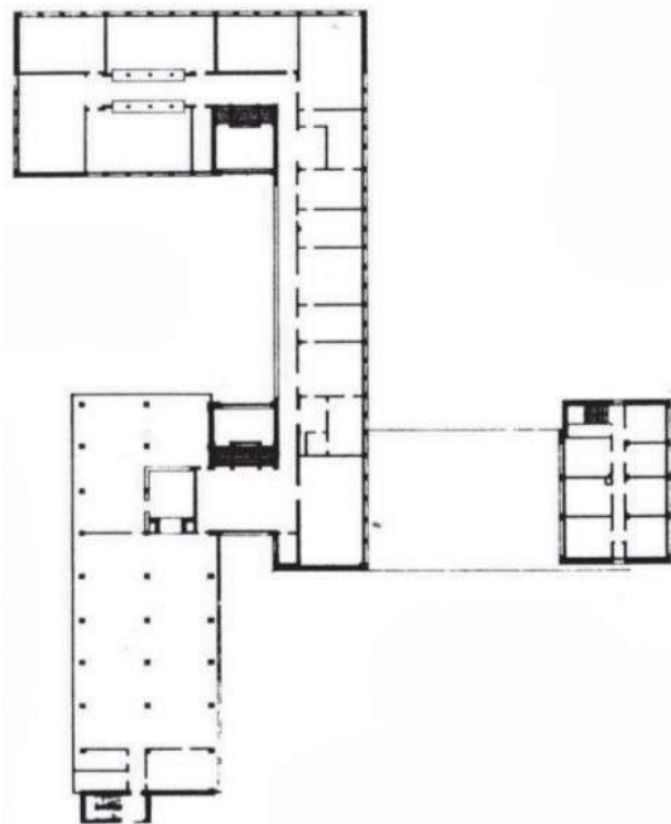
Bauhaus, Dessau – Planta do 1º pavimento
