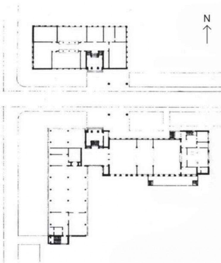
Bauhaus, Dessau – Planta do térreo
