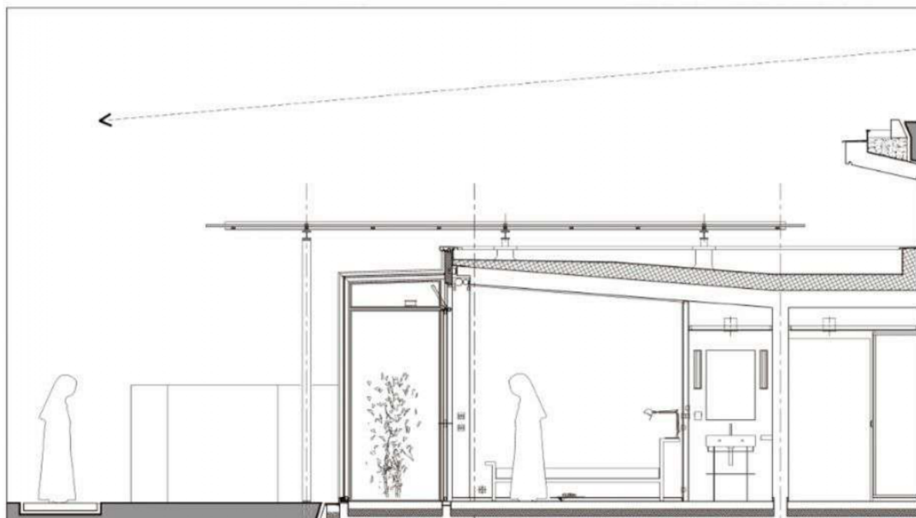
Corte dos anexos
