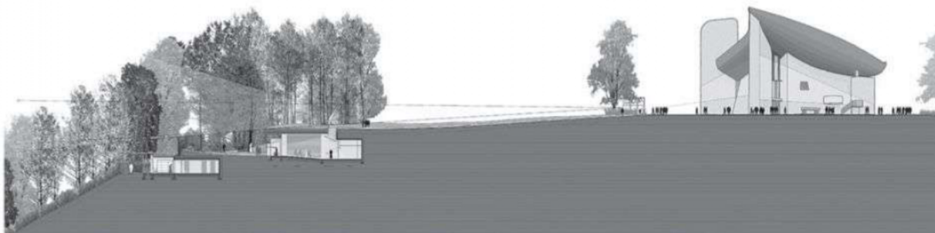
Corte de conjunto com a capela e Ronchamp e anexos
