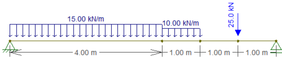
Figura 1: Viga submetida a carregamentos
