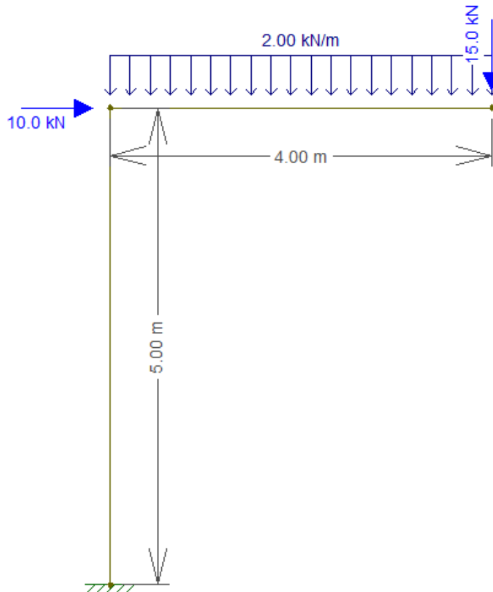
Figura 1: Pórtico submetido a carregamentos
