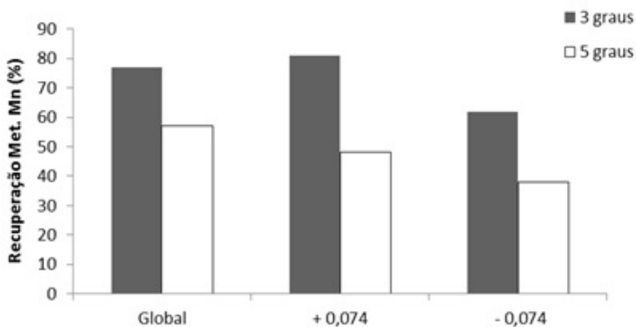
Figura 1 - Resultados dos testes em mesa oscilatória
