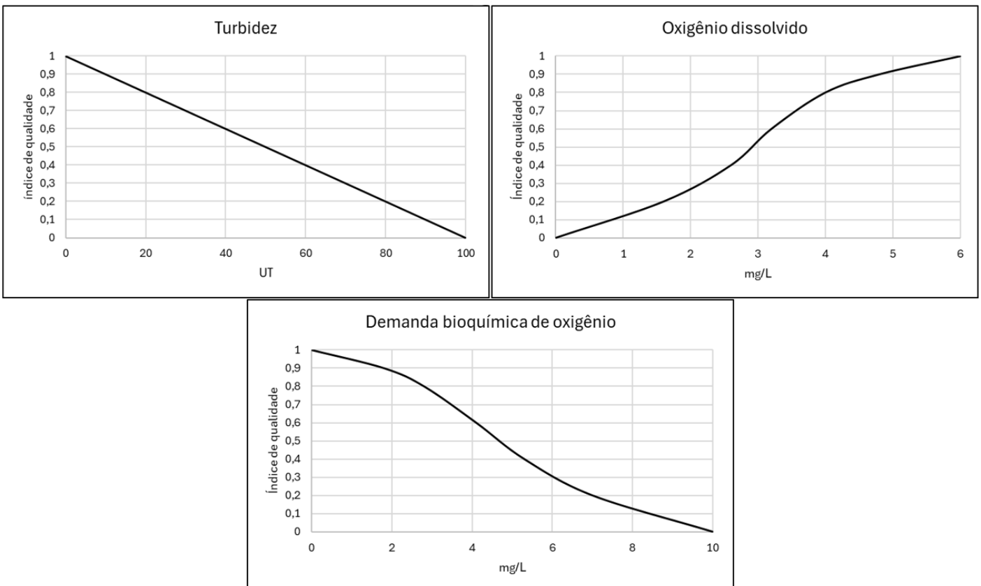
Figura 1 – Índices de qualidade ambiental para turbidez, oxigênio dissolvido e demanda bioquímica de oxigênio
