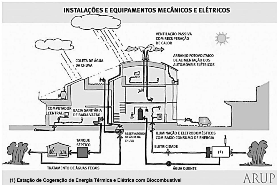
Figura 1. Diagrama dos sistemas de edificação sustentáveis de BedZED. Imagem © Arup
