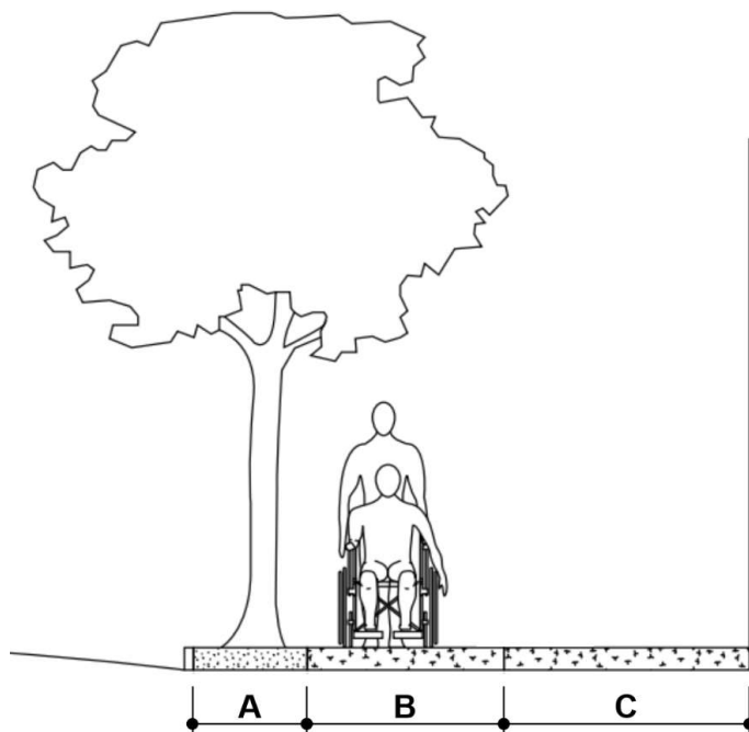
Figura 1. Faixas de uso da calçada – Corte (sem escala). Fonte: Editado a partir da ABNT NBR 9050:2020.
