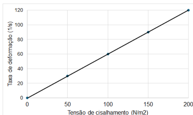
Figura 2 – Reograma da mistura Z na temperatura de 20^\circ\text{C}
