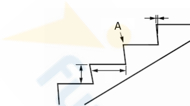
Figura 1 – Espelho inclinado Sem escada. Fonte: NBR 9050:2020.
