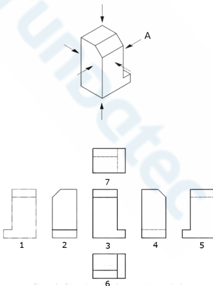
Figura 1 – Disposição das vistas no primeiro diedro Fonte: NBR 17006:2021.
