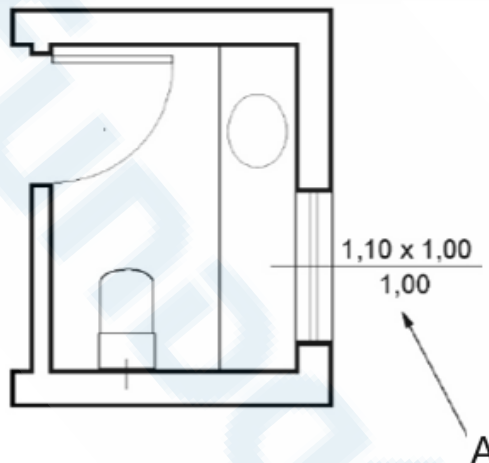
Figura 2 – Representação da designação de janelas Fonte: NBR 6492:2021.
