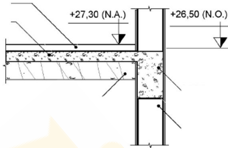
Figura 4 Sem escala. Fonte: NBR 6492:2021.
