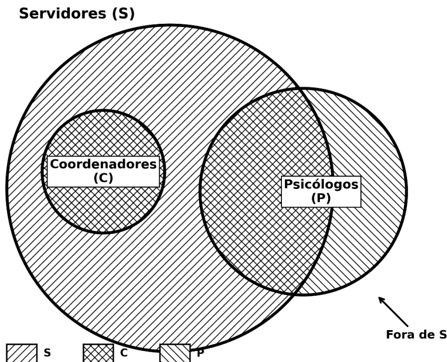
Figura 5 — Relações de inclusão e interseção entre os conjuntos.
