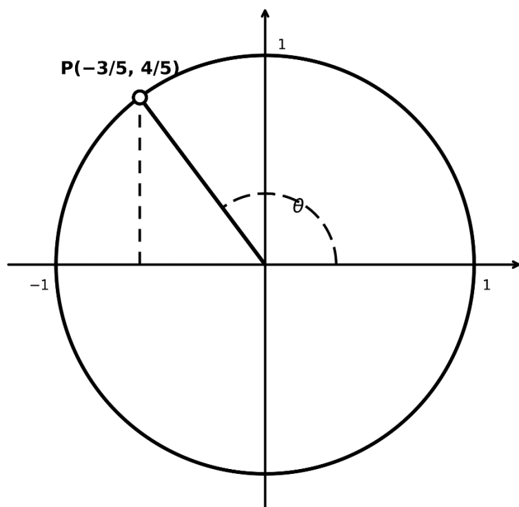
Figura 3 — Ponto P no ciclo trigonométrico unitário.
