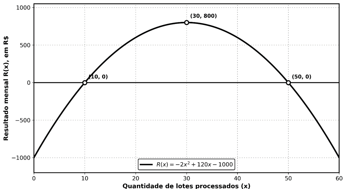
Figura 2 — Resultado mensal em função da quantidade processada.
