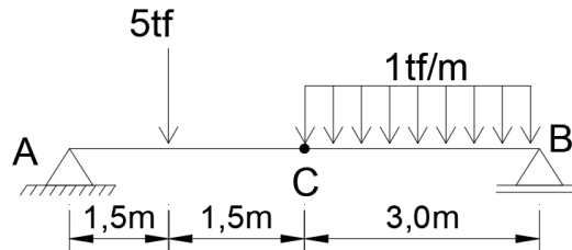
Figura 1 – Viga bi apoiada (fonte: autora)
